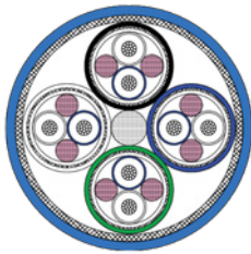
DVI
