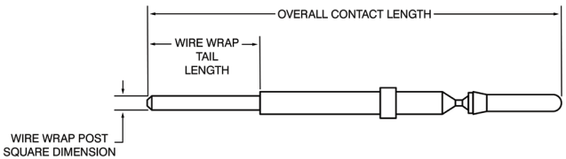
Wire Wrap Contact
